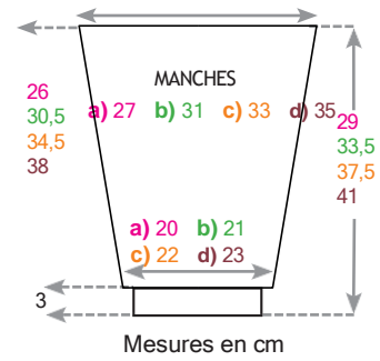
Mesures en cm
